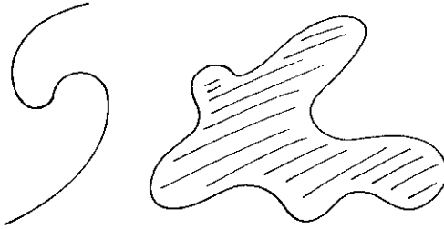
Abbildung 8.8: Kurve und Fläche
