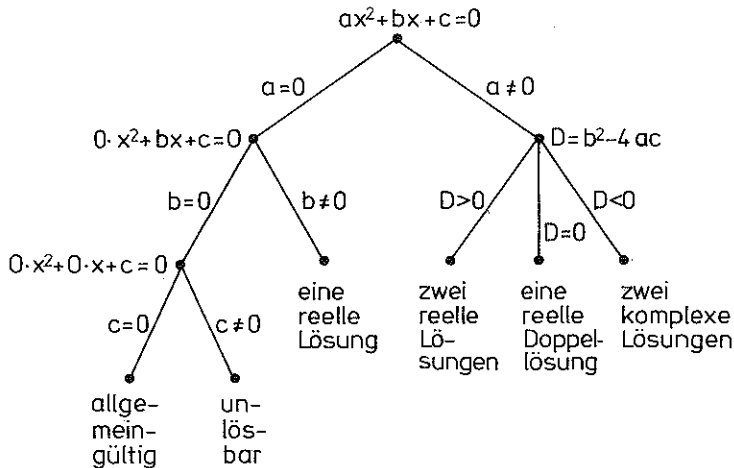
Abbildung 5.1: Fallunterscheidungen zur quadratischen Gleichung
